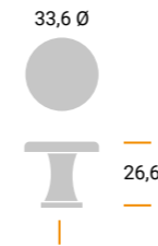
MZ2305 Materiale / Material: Metal Diam. / Diam.: 33,6 mm. Alt. / Height 26,6 mm. Interasse / Cd 0 mm.
