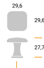
MZ2307 Materiale / Material: Metal Largh. / Width: 29,6 mm. Lungh. / Length 29,6 mm. Alt. / Height 27,7 mm. Interasse / Cd 0 mm.
