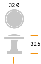
MZ2316 Materiale / Material: Metal Diam. / Diam.: 32 mm. Alt. / Height 30,6 mm. Interasse / Cd 0 mm.
